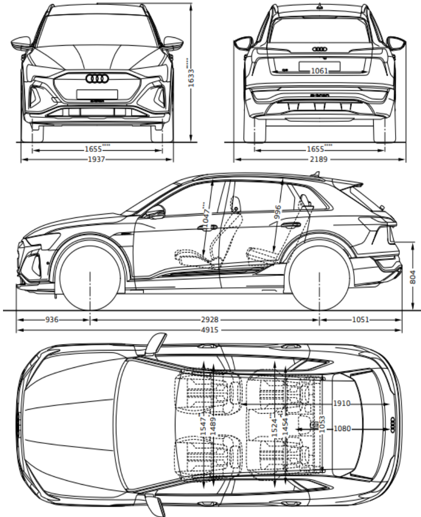
Audi Q8 e-tron
