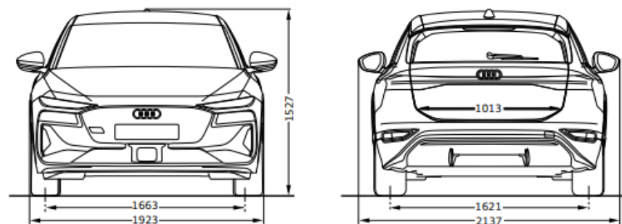
Audi S6 Avant e-tron
